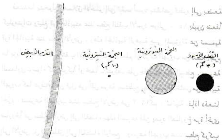
شكل ١٠.٣ النسبة بين أبعاد القزم الأبيض والنجمة النيوترونية والثقب الأسود ومقدار نصف قطر كل منهم
