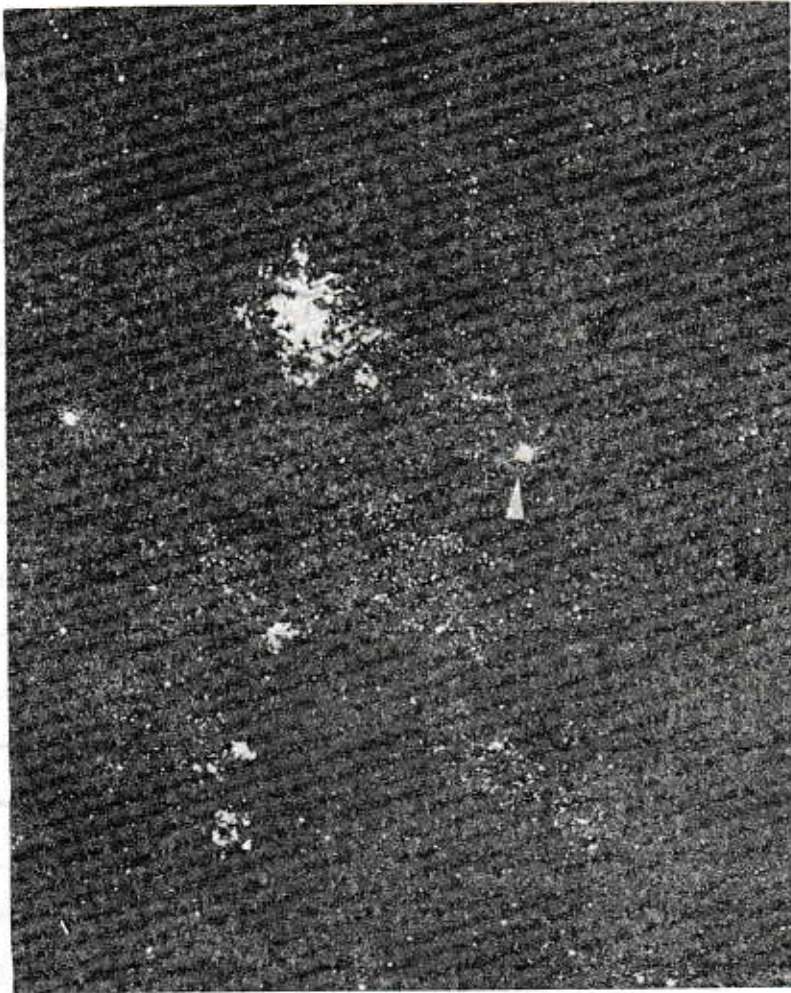
شكل ١٥.٣ الانفجار النجمي الأعظم الذي حدث سنة ١٩٨٧ يشير إليه سهم أبيض في هذه الصورة التي أخذت في ٢٥ فبراير ١٩٨٧ لسحب ماجلان التي تظهر في النصف الجنوبي للمكرة الأرضية من مرصد شبلي .
